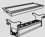
3 PC + 1 USB A 5v + 1 USB C 5v + 1 passage de câbles personnalisable
