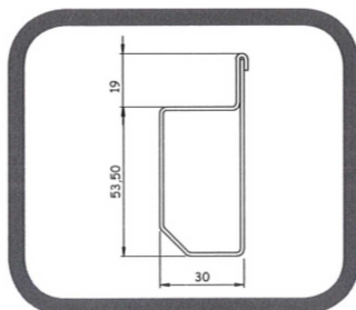
Coupe du longeron.
