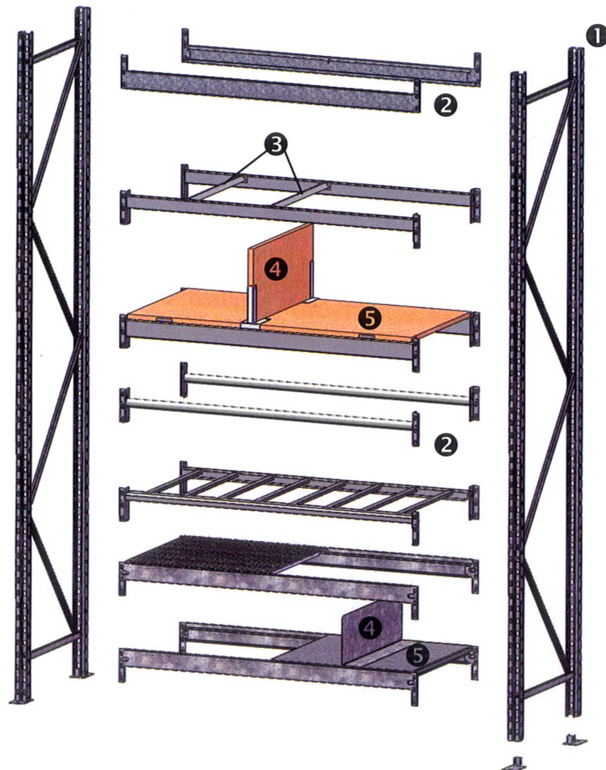
Assemblage longeron/montant (montant perforé au pas de 50 mm).
