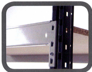
Assemblage longeron/montant (montant perforé au pas de 50 mm).
